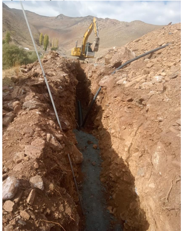
Tuzluca İlçesi Sarıbulak Köyü Kanalizasyon Fosseptik Çukuru Yapım İşi
